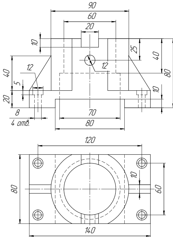
Кронштейн
