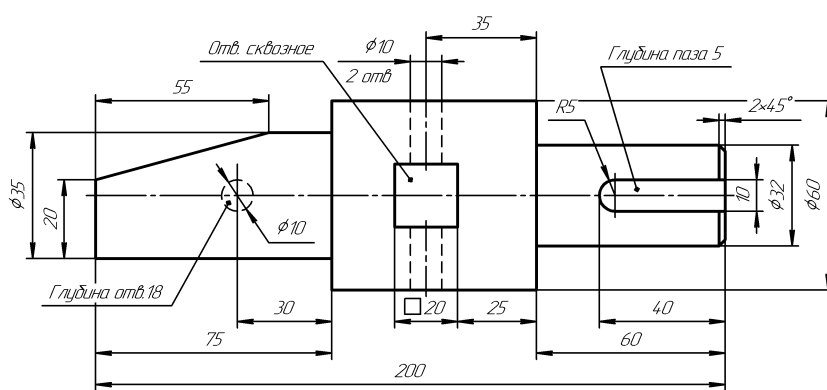
Вал
