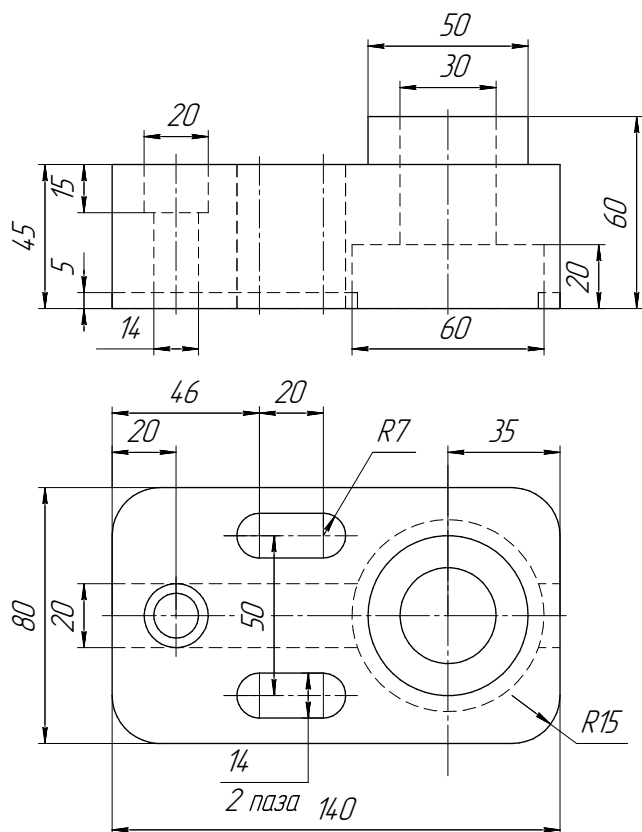
Плита
