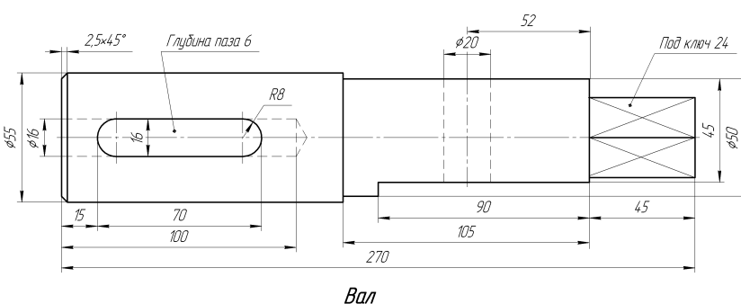
Вал
