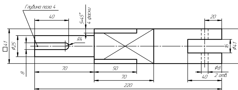
Вал
