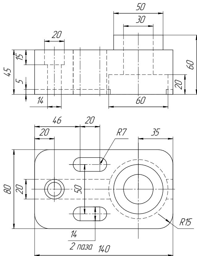
Плита
