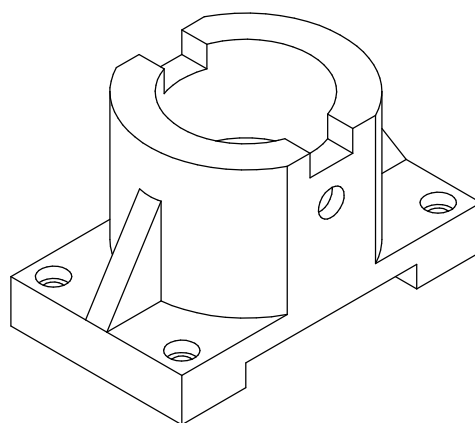
Кронштейн
