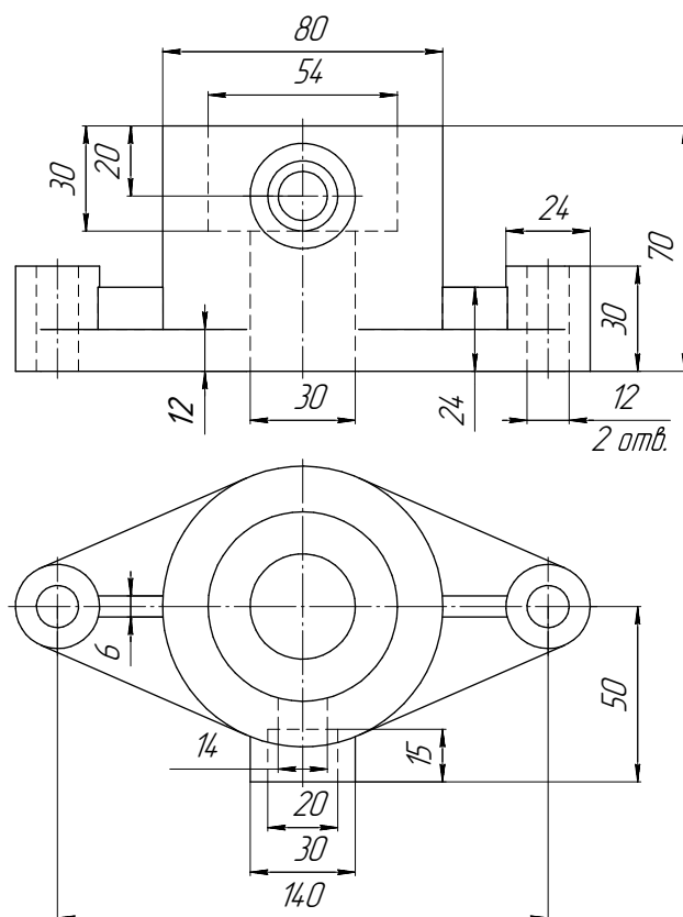
Корпус
